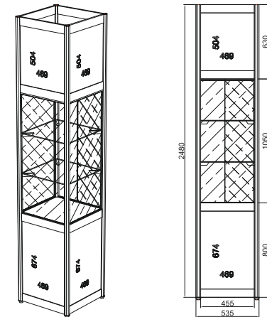
Витрина 500 x 500 x 2500 мм
