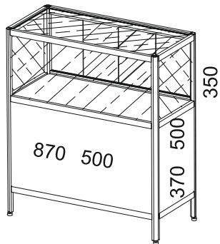
Витрина 940 x 430 x 1100 мм
