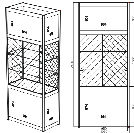
Витрина 1000 x 500 x 2500 мм
