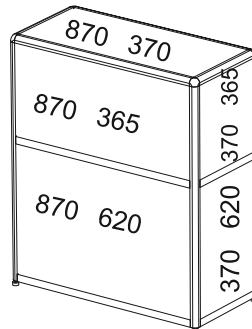
Информационная стойка 940 x 430 x 1100 мм
