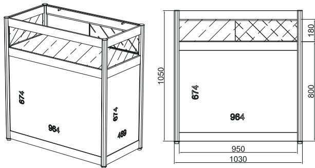
Витрина 1000 x 500 x 1000 мм
