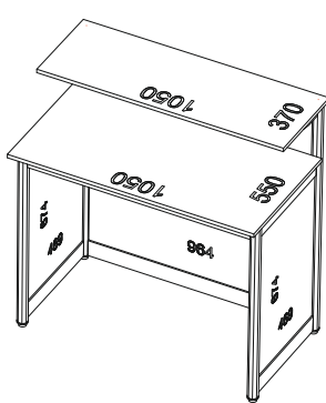
Барная стойка со столешницей 1000 x 500 x 1000 мм
